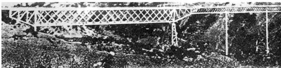
Η παλαιά γέφυρα Παπαδιάς στον Σκαμνό.
