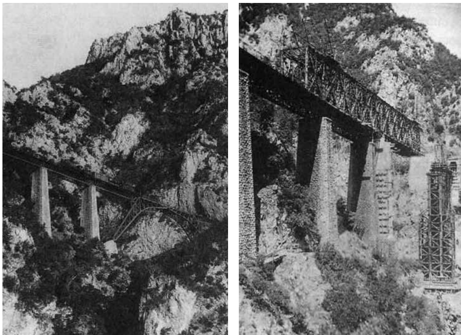
Η γέφυρα Ασωπού καταστράφηκε στις 21.06.1943 με μια από τις πιο εντυπωσιακές επιχειρήσεις δολιοφθοράς στο Β' Παγκόσμιο Πόλεμο. Αριστερά, η γέφυρα όπως πρωτοκατασκευάστηκε στις 20.07.1905. Αν και η γέφυρα κατασκευάστηκε εκ νέου (δεξιά), κατέρρευσε και πάλι, σκοτώνοντας 40 Έλληνες και Γερμανούς.
