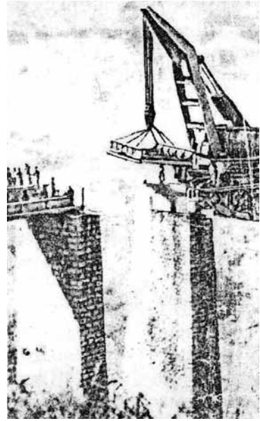
Μετά την ανατίναξη, οι Γερμανοί προχωρούν στην ανακατασκευή της γέφυρας του Γοργοπόταμου.
